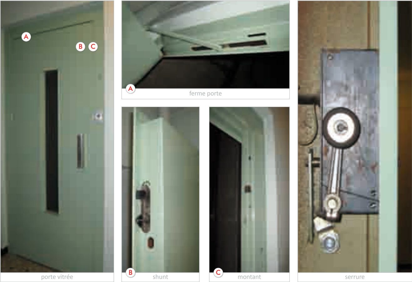
ex : serrure droite sur porte OTIS PILO
