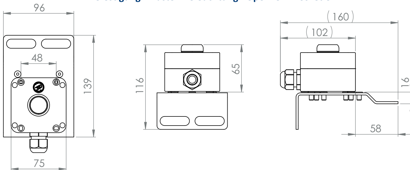
Fixation + Boîtier éclairage - Fastening + lighting unit Befestigung + Kasten Beleuchtung - Upevnení + osvetlení
