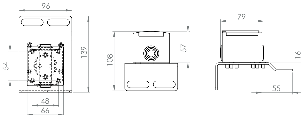
Fixation + Boîtier prise courant - Fastening + power socket unit Befestigung + Kasten Steckdosen - Upevnení + zásuvky
